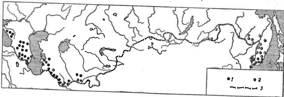
Рис. 18. Распространение леопарда в СССР.
